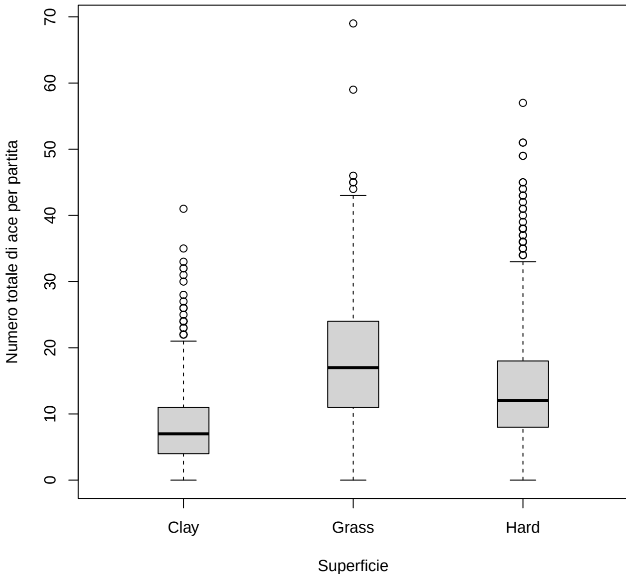
Diagramma a scatola e baffi di tot_ace condizionato a surface
